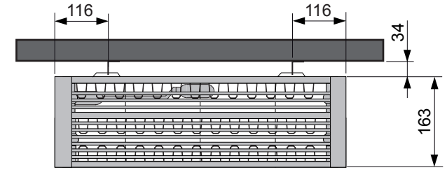
Bovenaanzicht Type 33
