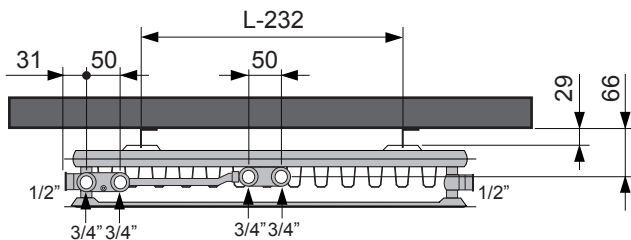
Onderaanzicht Type 21S
