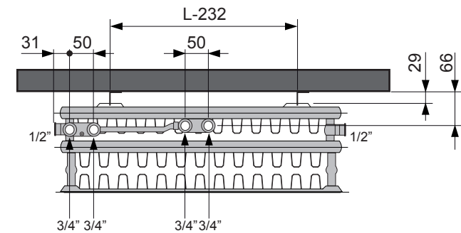
Onderaanzicht Type 33
