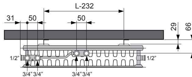
Onderaanzicht Type 22
