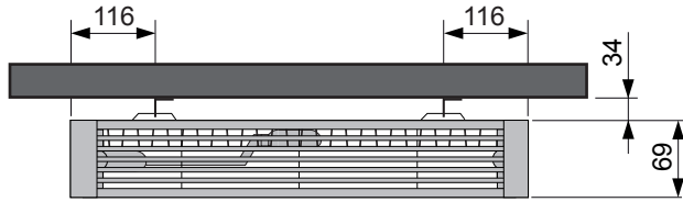
Bovenaanzicht Type 21S
