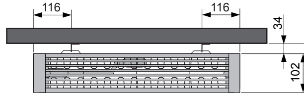
Bovenaanzicht Type 22
